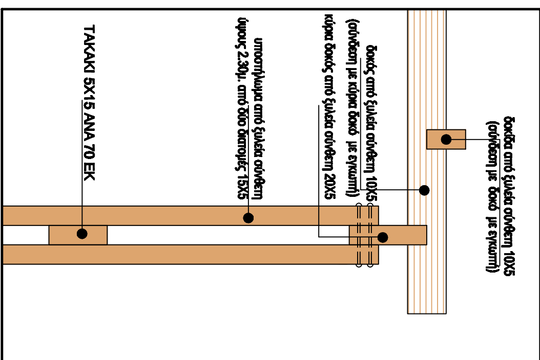
ΑΕΤΟΤΗΡΕΙΑ ΚΥ, 1:10
